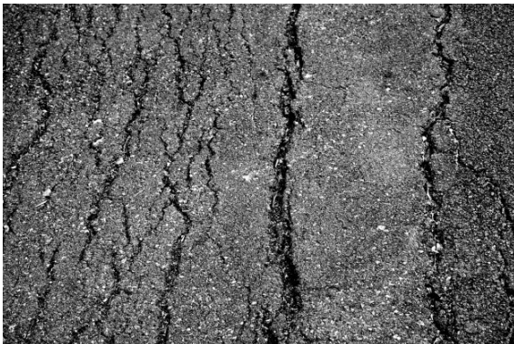
Asphalte (goudron)
